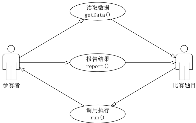
图 6 参赛者用例
